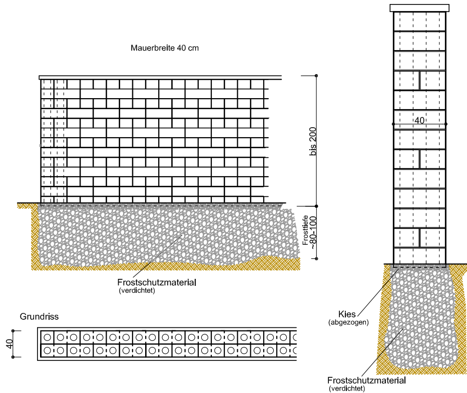
Freistehende Mauer bis 200 cm Höhe bei 40 cm Breite
