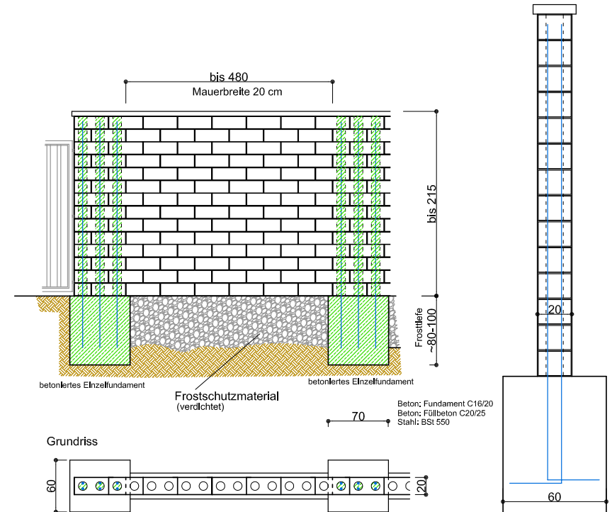
Freistehende Mauer bis 215 cm Höhe bei 20 cm Breite
