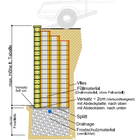
Stützmauer mit Ankerblock (3 Reihen)
